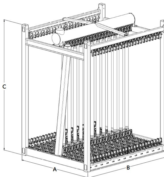
Cassetta LEAPmbr da 52 moduli
